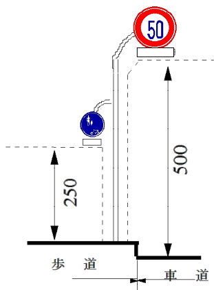
図例(3) オーバー・ハング方式
