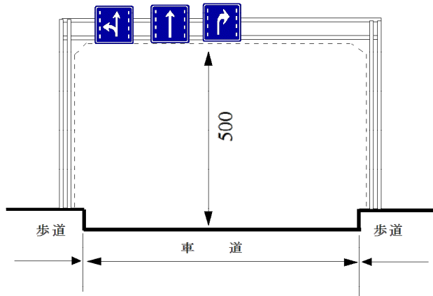
図例(2) オーバー・ヘッド方式
